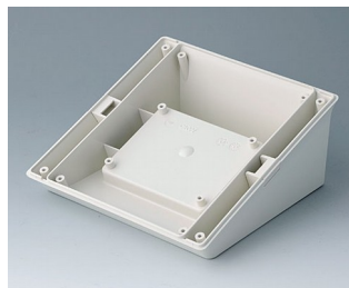
B4044827 Socle M - pupitre - ABS (UL 94 HB) gris blanc RAL 9002 153x153x63mm
