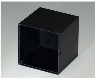
A8025251 BOITIER VIDE POUR MODULES, Vers. I PF (UL 94 V-0) noir RAL 9005 25x25x25mm
