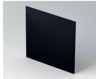
B6134221 Plaque avant PPO (UL 94 V-0) noir RAL 9005 90,7x90,7x2mm
