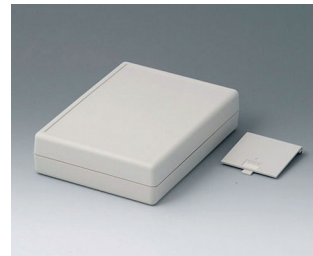
A9413757 BOITIER COQUILLES G 190, Vers. V ABS (UL 94 HB) gris blanc RAL 9002 138x190x45,5mm
